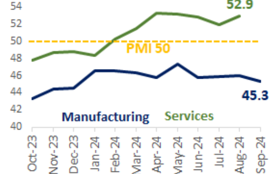
EU PMI
